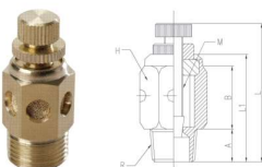
MODEL(ØD-T) Tube(Metric)–Thread(R)
