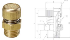
MODEL(ØD-T) Tube(Metric)–Thread(R)
