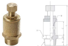
MODEL(ØD-T) Tube(Metric)–Thread(R)
